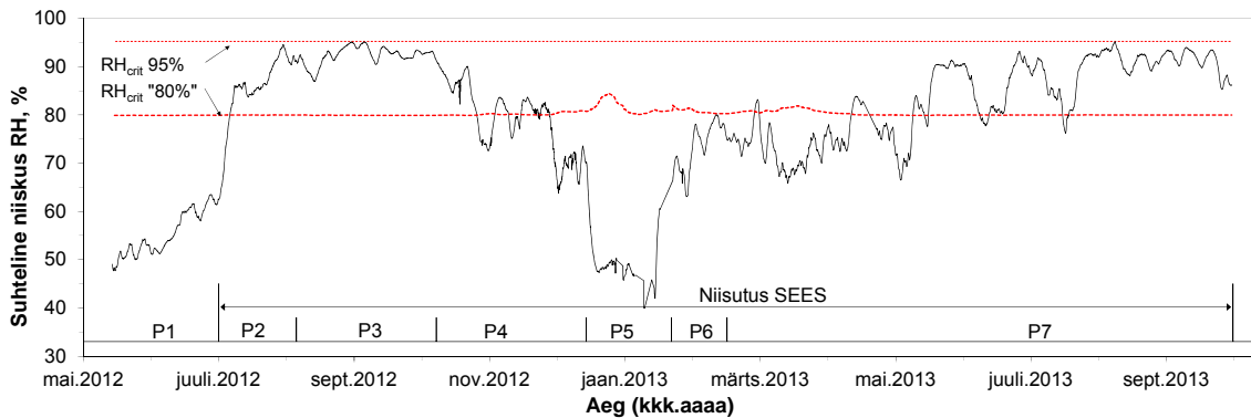
Joonis 14 Suhteline niiskus soojustuse CaSi ja esialgse seina vahel; niisutusperiodid.
