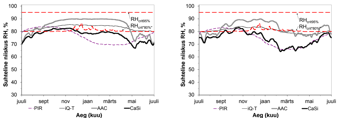
Joonis 22 Arvutustulemused – suhtelised niiskused soojustussüsteemide taga ühe aasta jooksul pärast stabiilse seisundi saavutamist, niiskuslisa \Delta v=6\text{ g/m}^3 Vasakul: Eesti hallituse testaasta tingimustes Paremal: Eesti kondenseerumise testaasta tingimustes
