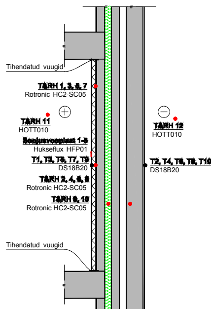
Joonis 6 Andurite paigutus seinas, vaade ja lõige testseintest.
