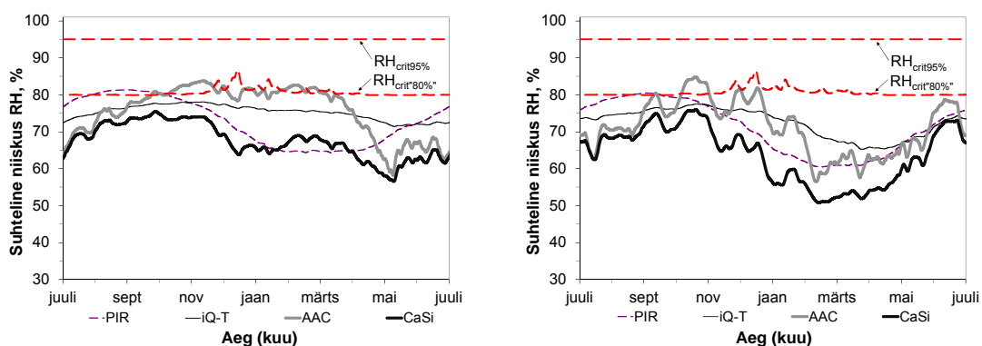
Joonis 21 Arvutustulemused – suhtelised niiskused soojustussüsteemide taga ühe aasta jooksul pärast stabiilse seisundi saavutamist, niiskuslisa \Delta v=4\text{ g/m}^3 Vasakul: Eesti hallituse testaasta tingimustes Paremal: Eesti kondenseerumise testaasta tingimustes
