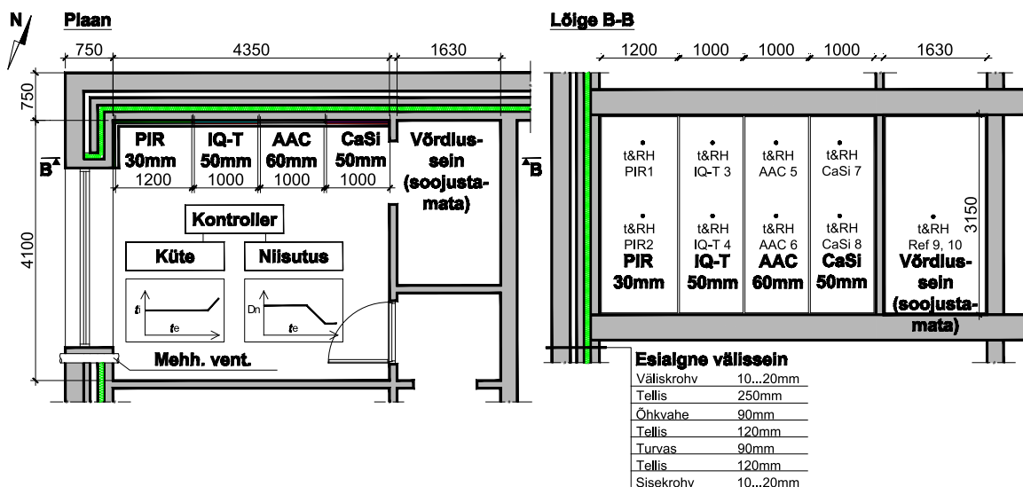
Joonis 5 Katseseina plaan ja lõige.
